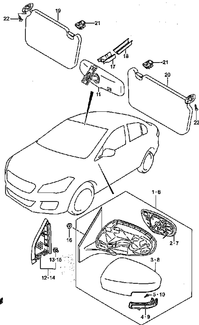
MIRROR/SUNVISOR
