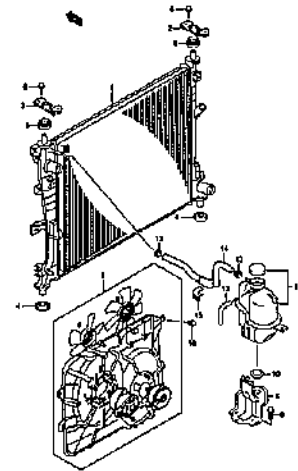
RADIATOR (3)
