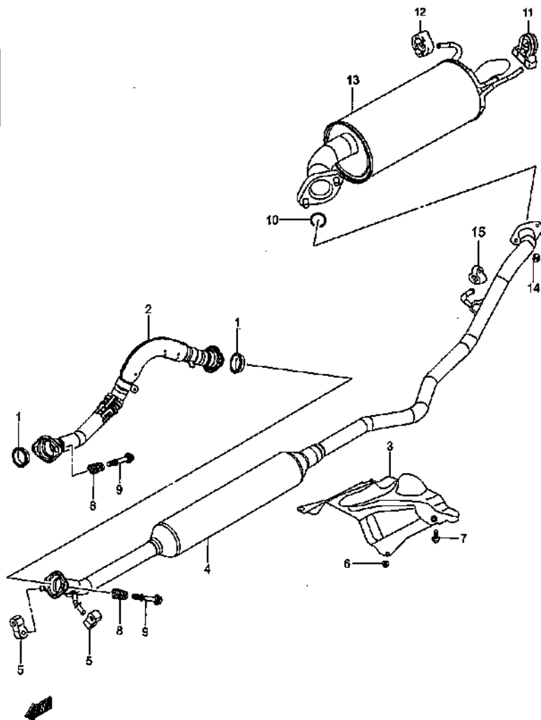
MUFFLER (2)
