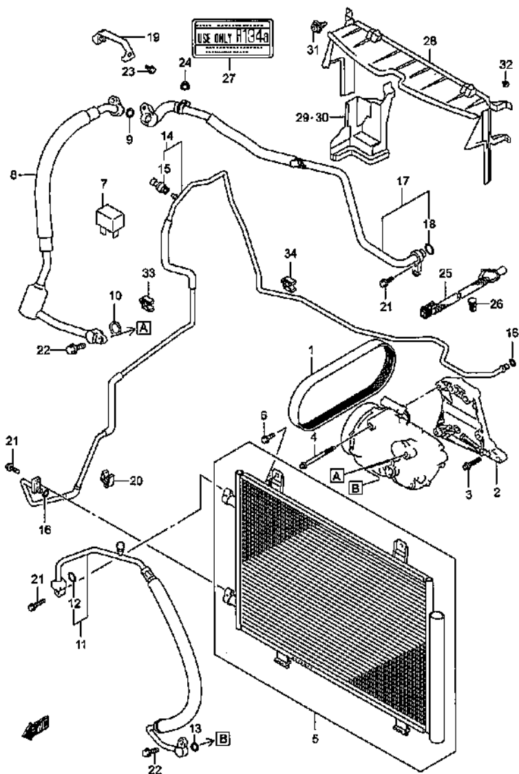
AIR CONDITIONER (2)
