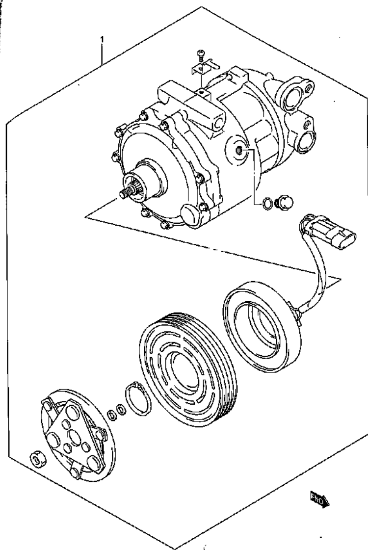
COMPRESSOR (2)
