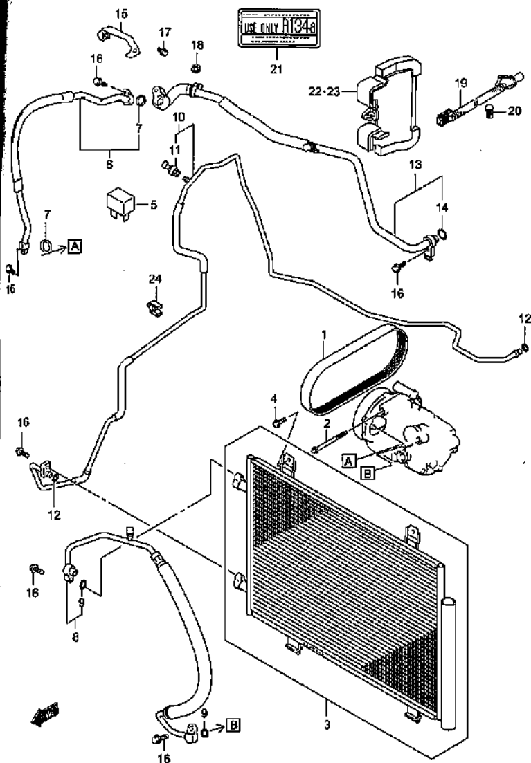
AIR CONDITIONER (2)
