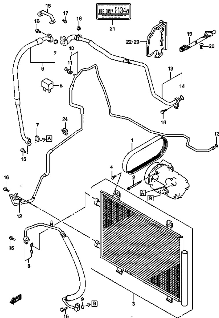
AIR CONDITIONER (1)
