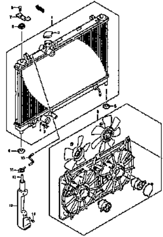
RADIATOR (2)
