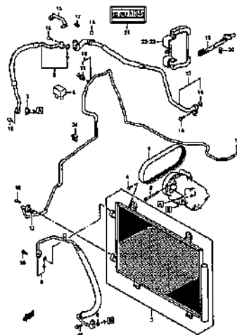
AIR CONDITIONER (2)
