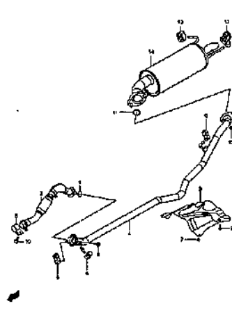
MUFFLER (2)
