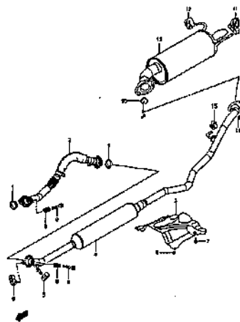
MUFFLER (2)
