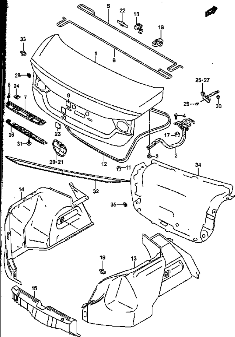
TRUNK LID
