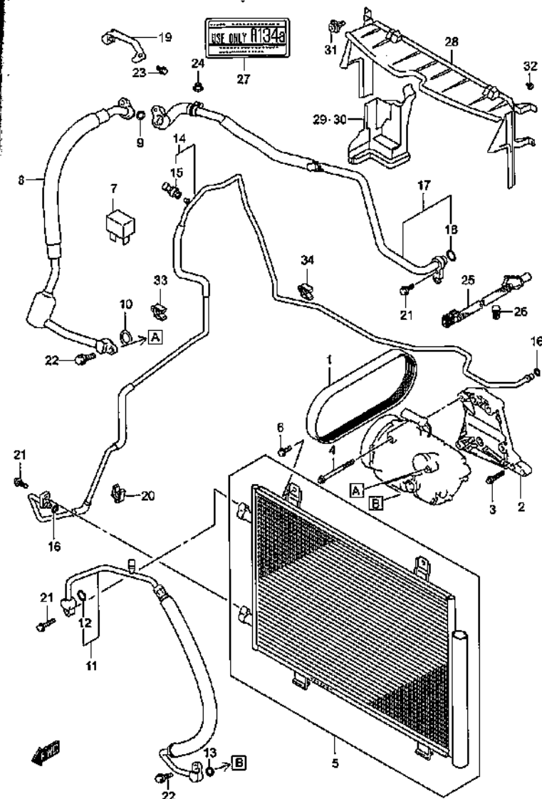
AIR CONDITIONER (2)
