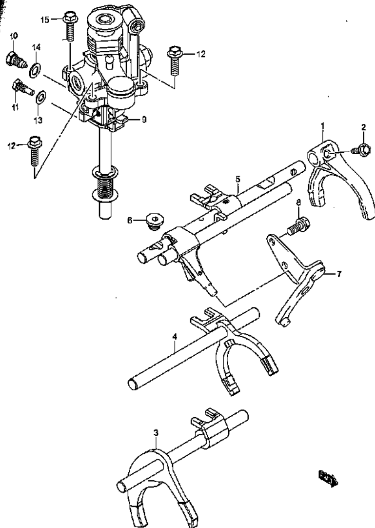
MT GEAR SHIFT FORK (2)
