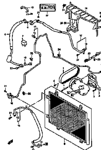
AIR CONDITIONER (2)
