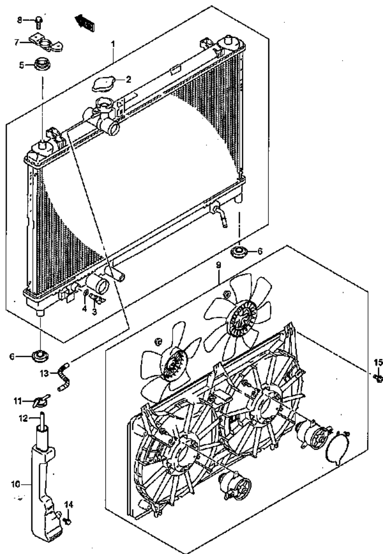
RADIATOR (1)
