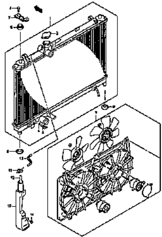
RADIATOR (1)
