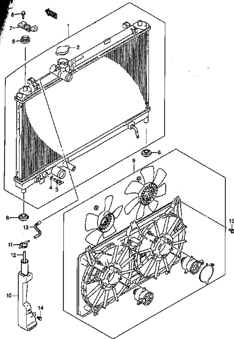
RADIATOR (2)
