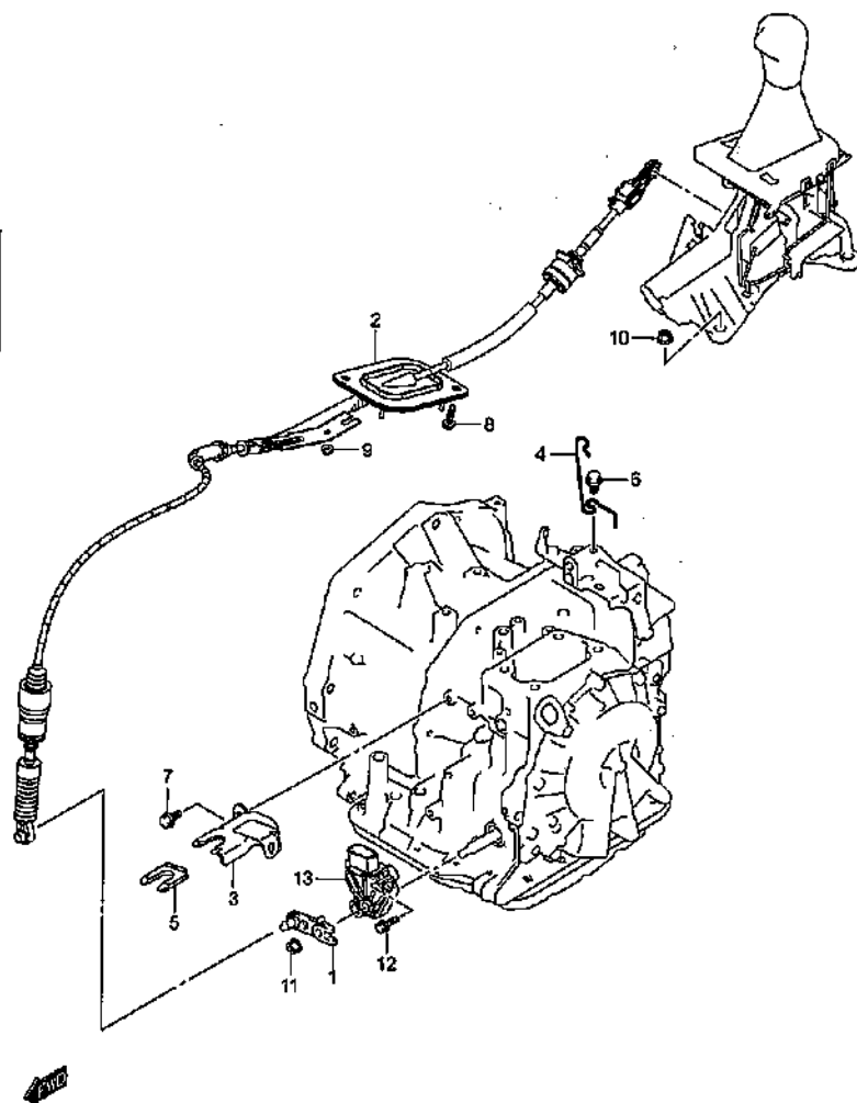
GEAR SHIFT CONTROL (3)
