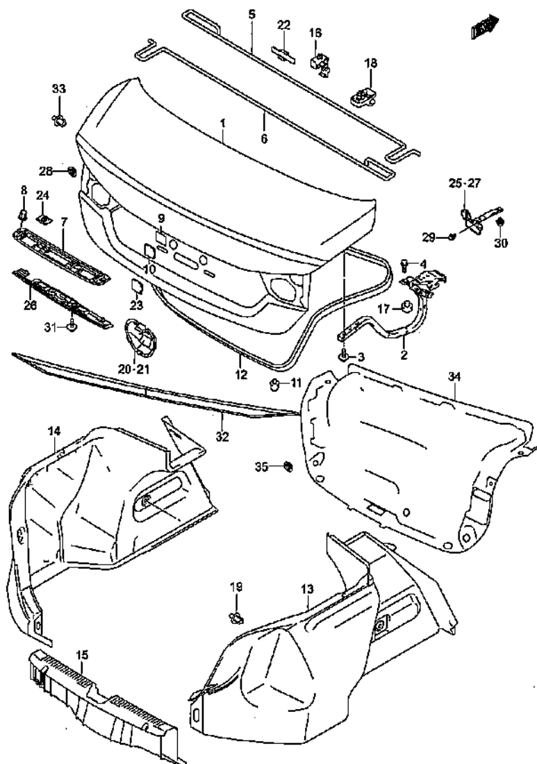
TRUNK LID
