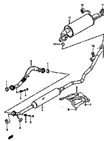
MUFFLER (1)
