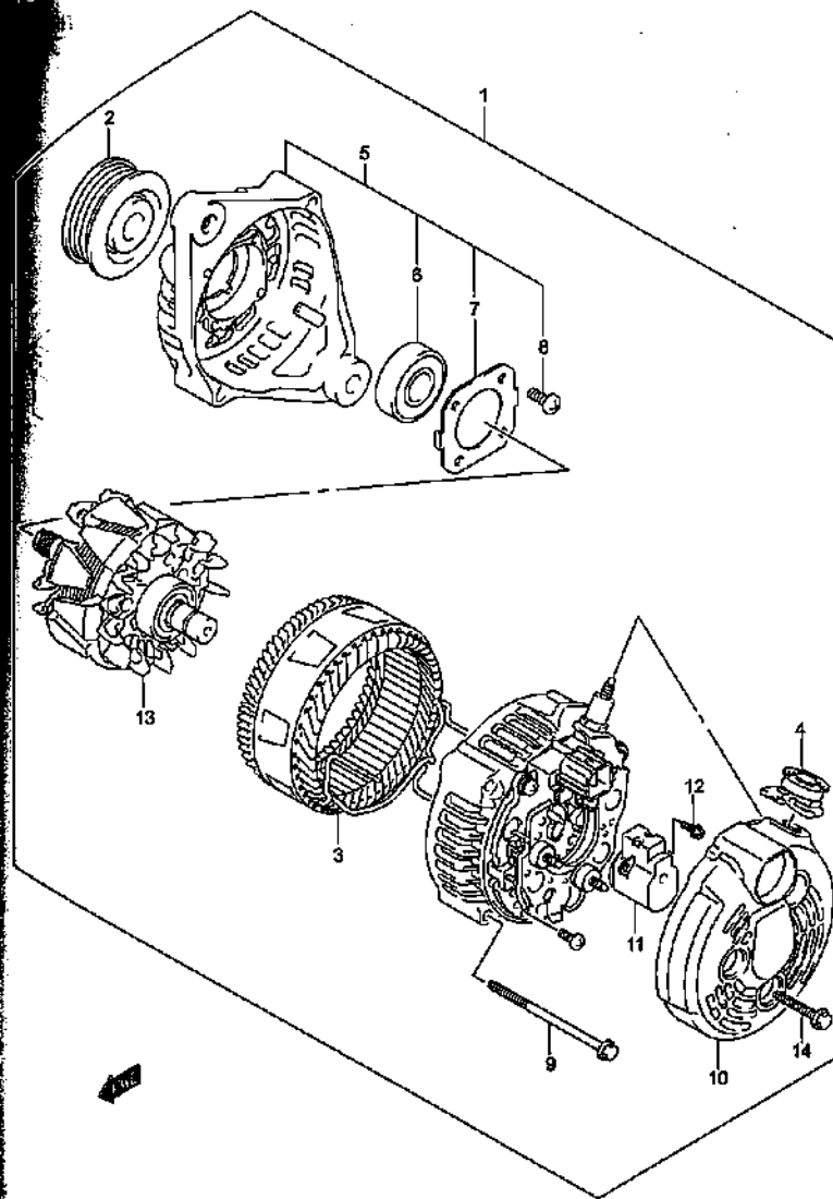
GENERATOR (2)
