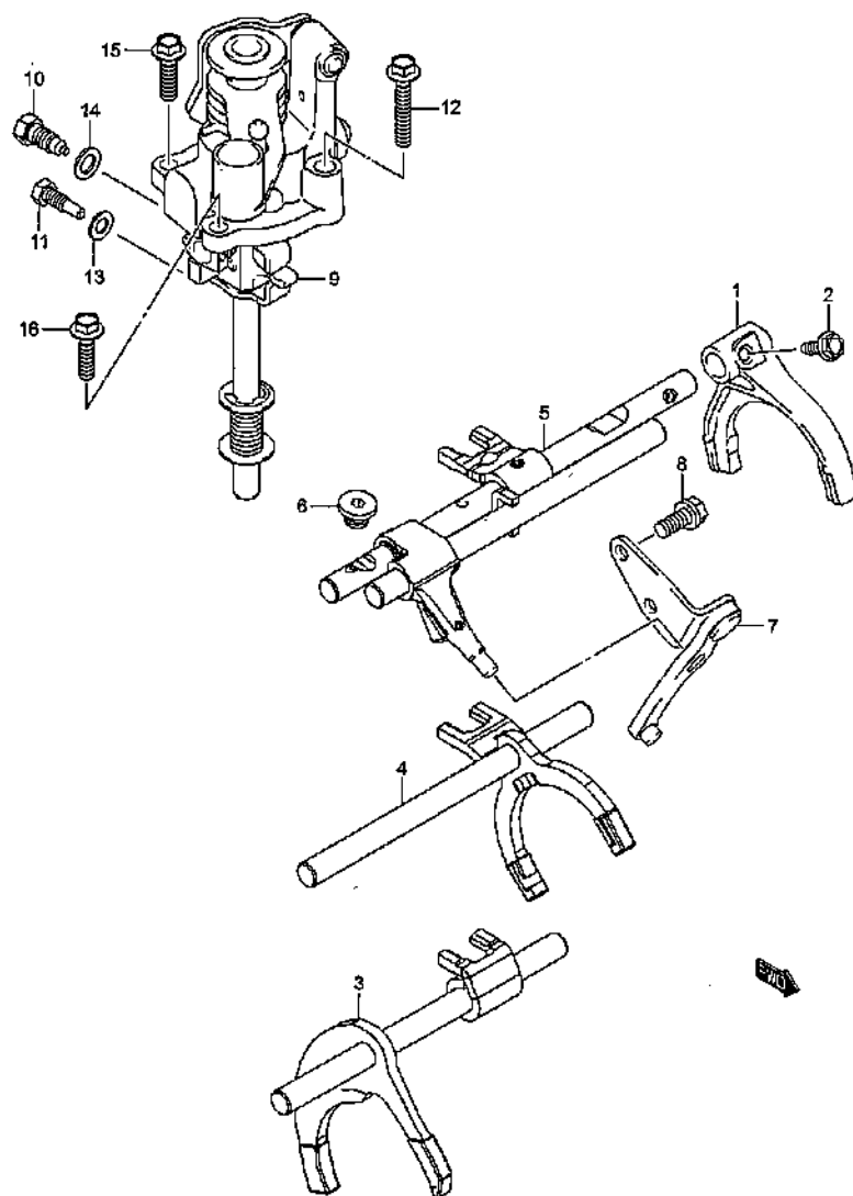
MT GEAR SHIFT FORK (1)
