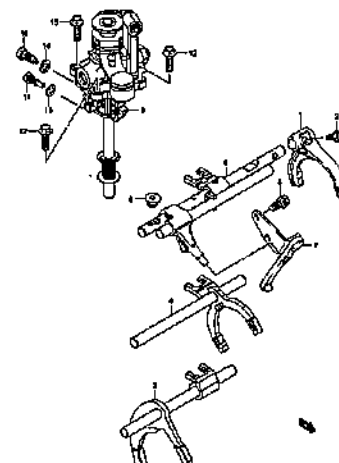
MT GEAR SHIFT FORK (2)
