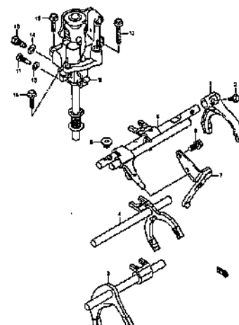
MT GEAR SHIFT FORK (1)
